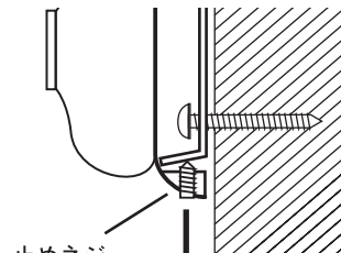
止めネジ
