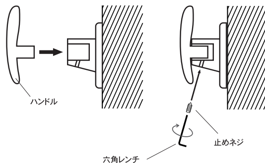
六角レンチ
